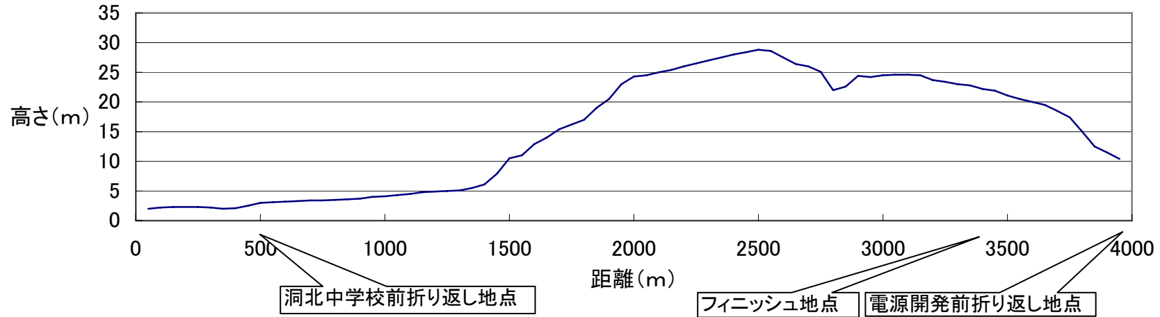
竹並バイパス高低表
